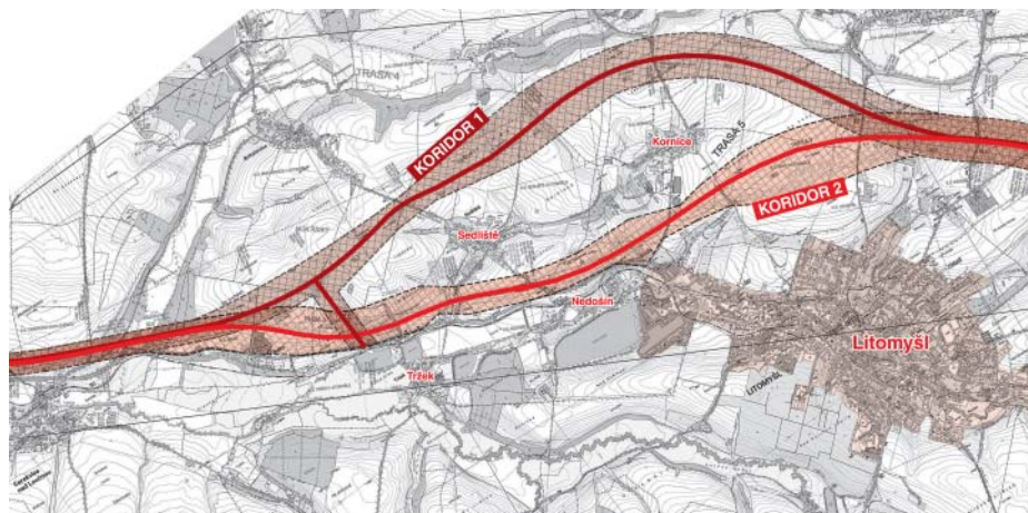
Dvě varianty rychlostní komunikace R35 u Litomyšle.
